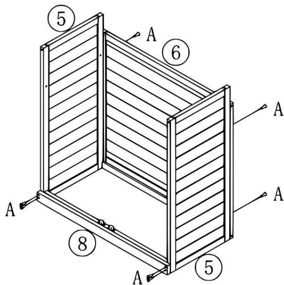
Krok 1 | A 3,5x40 mm (8)
