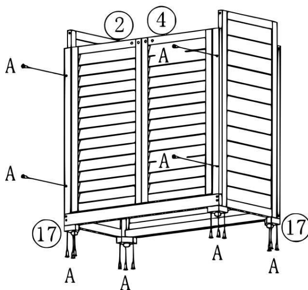
Krok 2 | A 3,5x40 mm (16)
